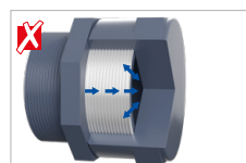
Aplicación tapón r/h tradicional con cinta PTFE. Traditional r/t plug application with PTFE.
