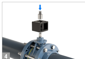
4 Instalar la torreta adaptador del motor y conexión eje motor. Install the actuator support adapter and the actuator shaft connection.
