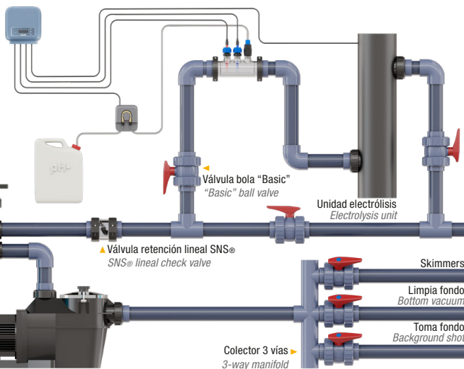
Ejemplo instalación Te SNS® visor portasondas con conexión sonda 1/2". Pg 136.
