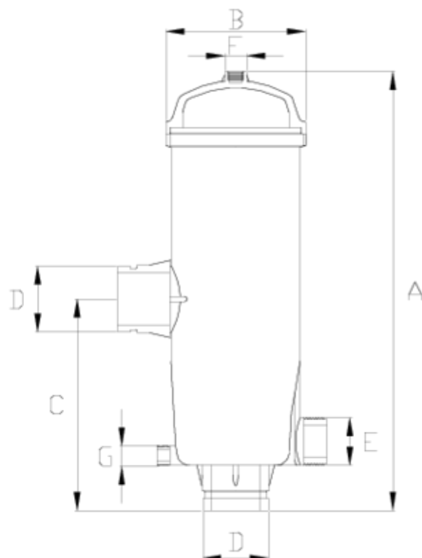
ITEM 803 | Filtro de cilindro perforado salida Netvitc® super
