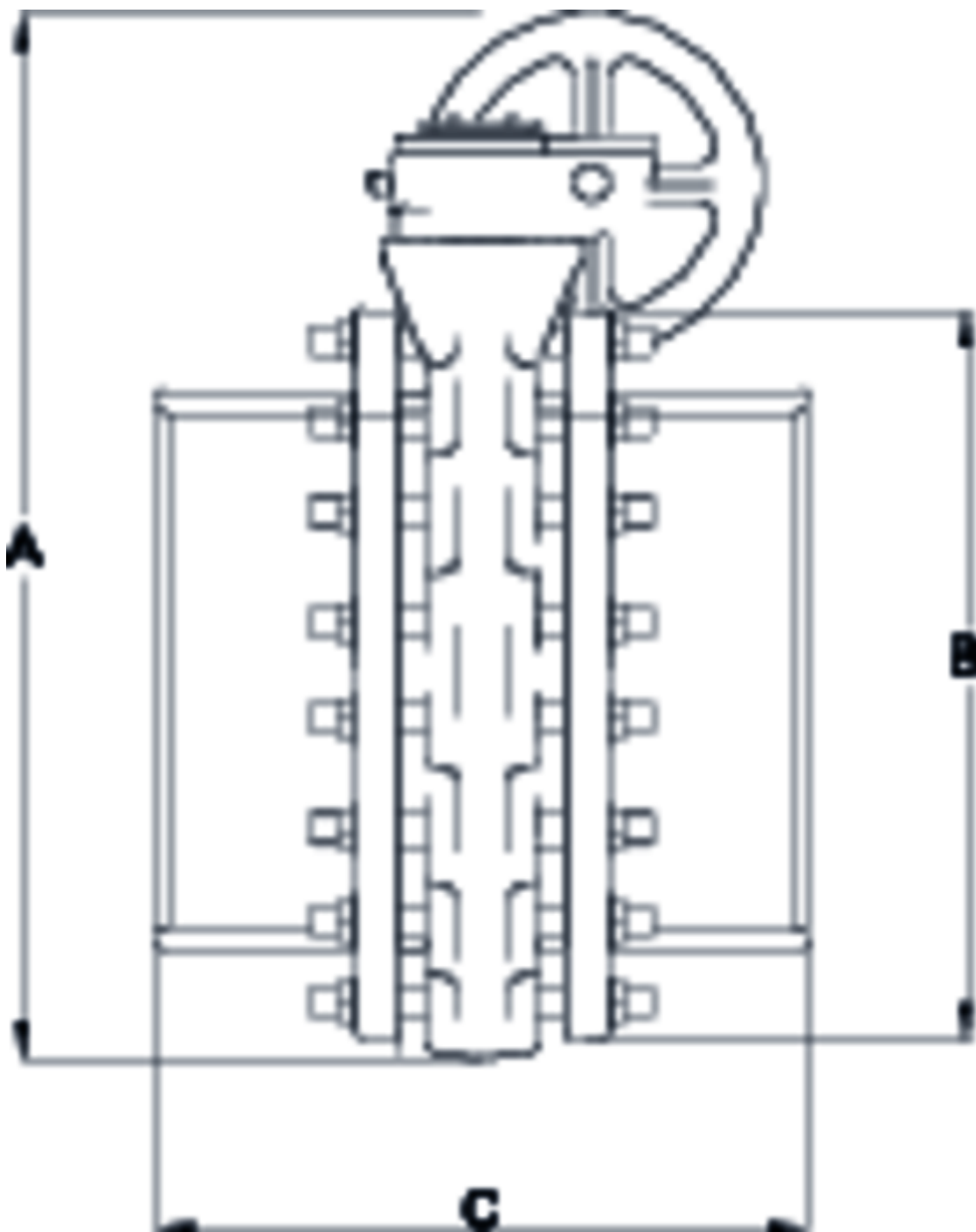
ITEM 187XL | Válvula de mariposa Implex bridas manoreductor 355
